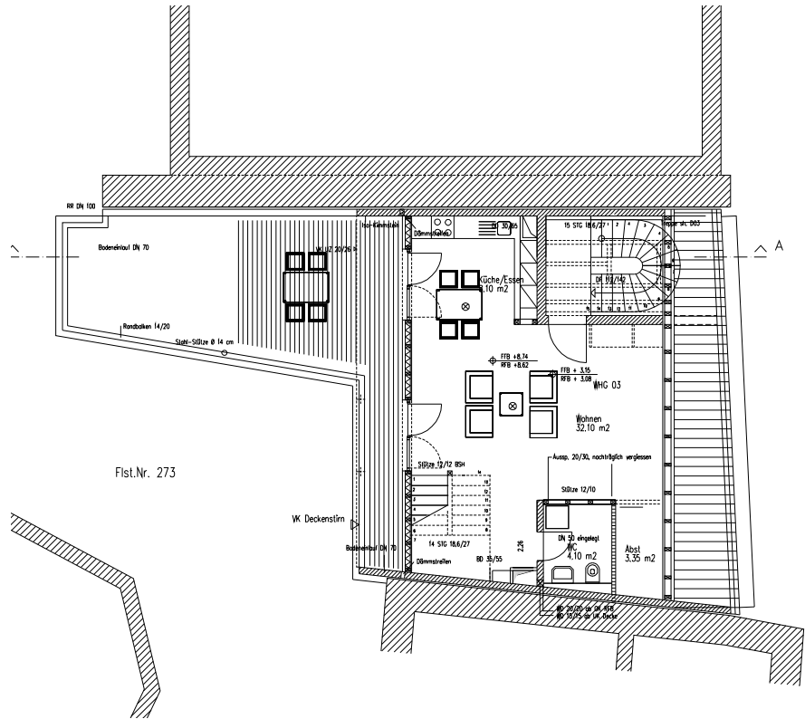
Grundriss 1.DG
