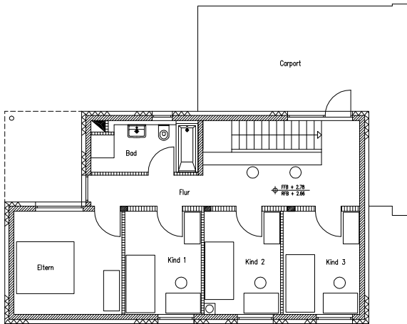
Grundriss Obergeschoss
