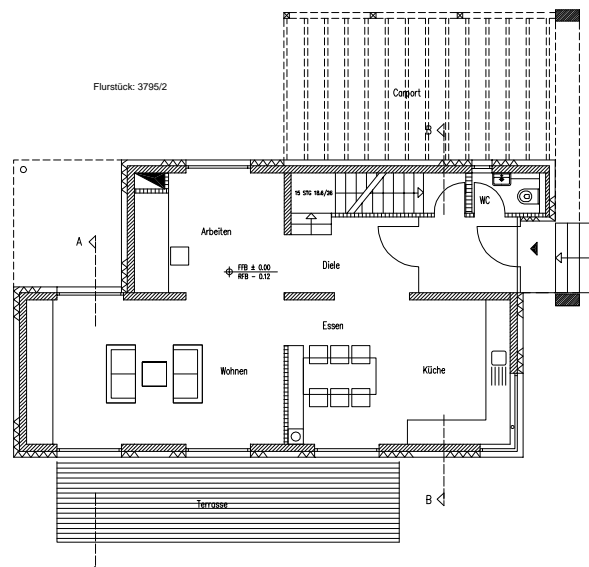
Grundriss Erdgeschoss
