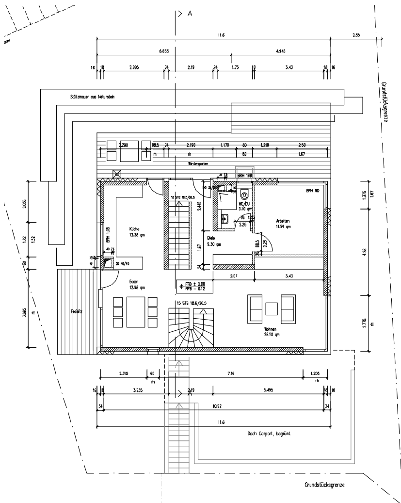
Grundriss Erdgeschoss
