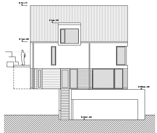
Ansicht Nordost
