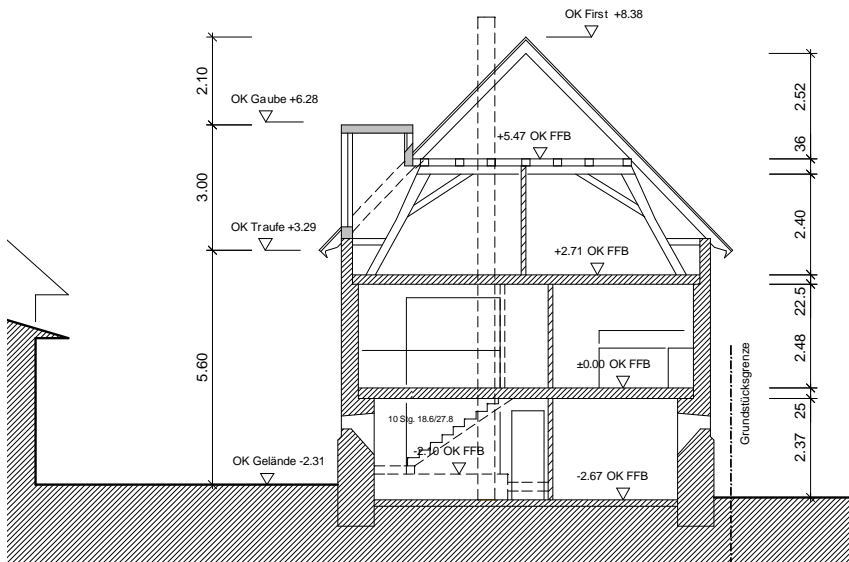
Schnitt A-A
