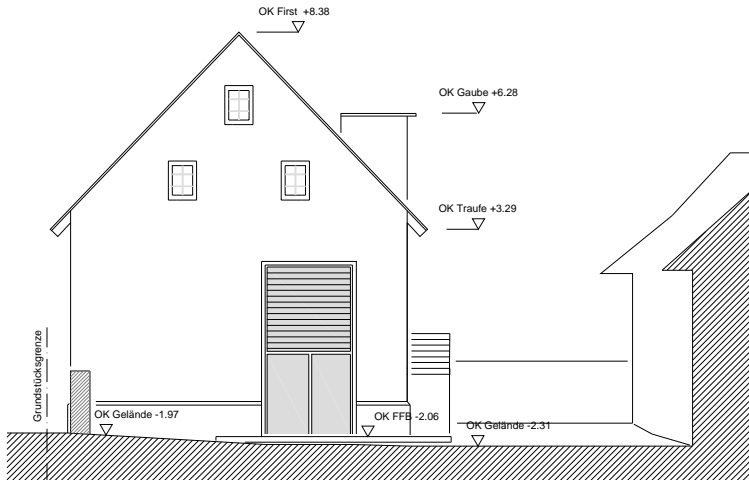
Ansicht Nordwest
