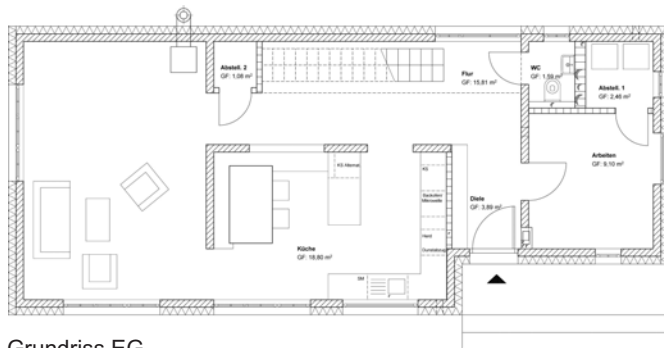
Grundriss EG
