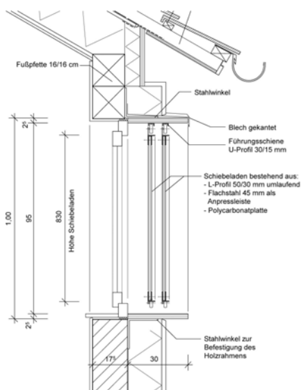
Detail Schiebeladen
